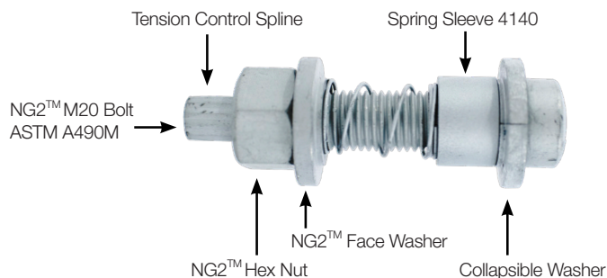
NG2™ Hex Nut A194 2H
